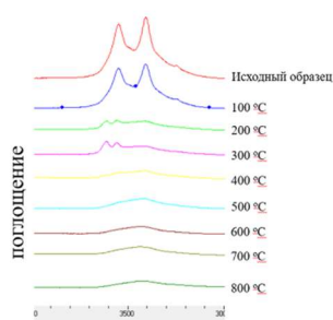
Рис. 6. ИК-спектры гипсоволокна в диапазоне от 4000 до 3000 \text{см}^{-1}
