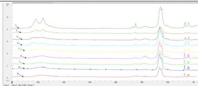
Рис. 5. ИК-спектры материала на основе гипса: 1 – исходный образец; 2-9 – обожженные образцы: 2 – 100 °C; 3 – 200 °C; 4 – 300 °C; 5 – 400 °C; 6 – 500 °C; 7 – 600 °C; 8 – 700 °C; 9 – 800 °C.
